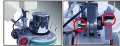
각도조절레버 핸드스크류 각도조절레버 레버를 앞으로 누르면 손잡이 각도 조절이 가능하고 뒤로 젖히면 고정됩니다.
